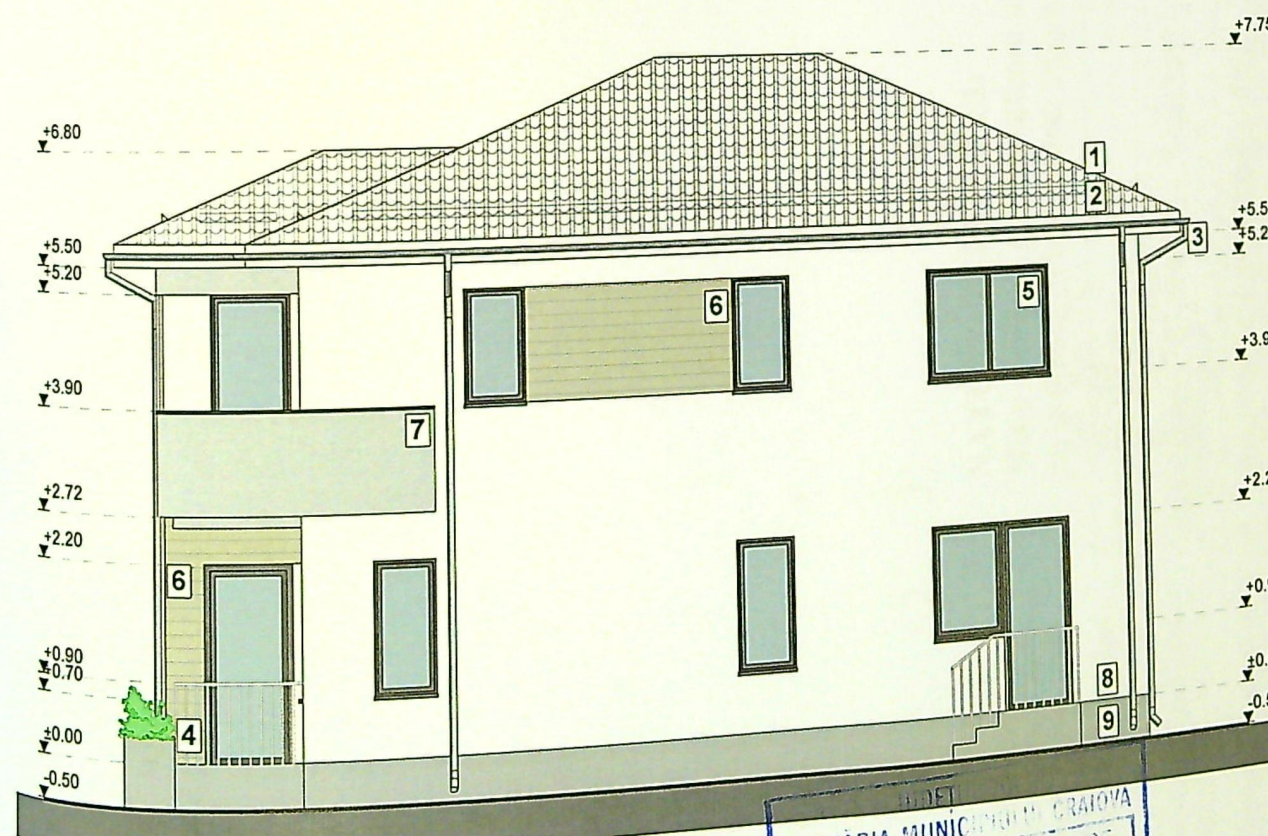
FATADA LATERALA DREAPTA
